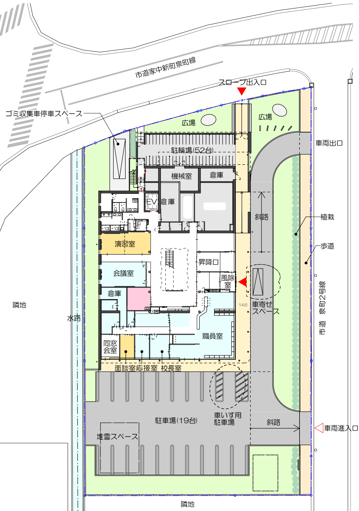
配置図・1階平面図
